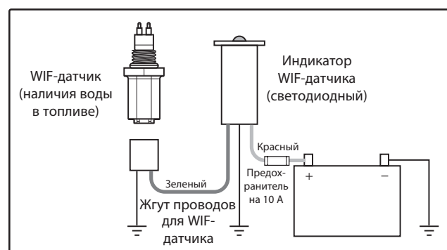
Рис. 2 – Схема электрических соединений WIF-датчика
